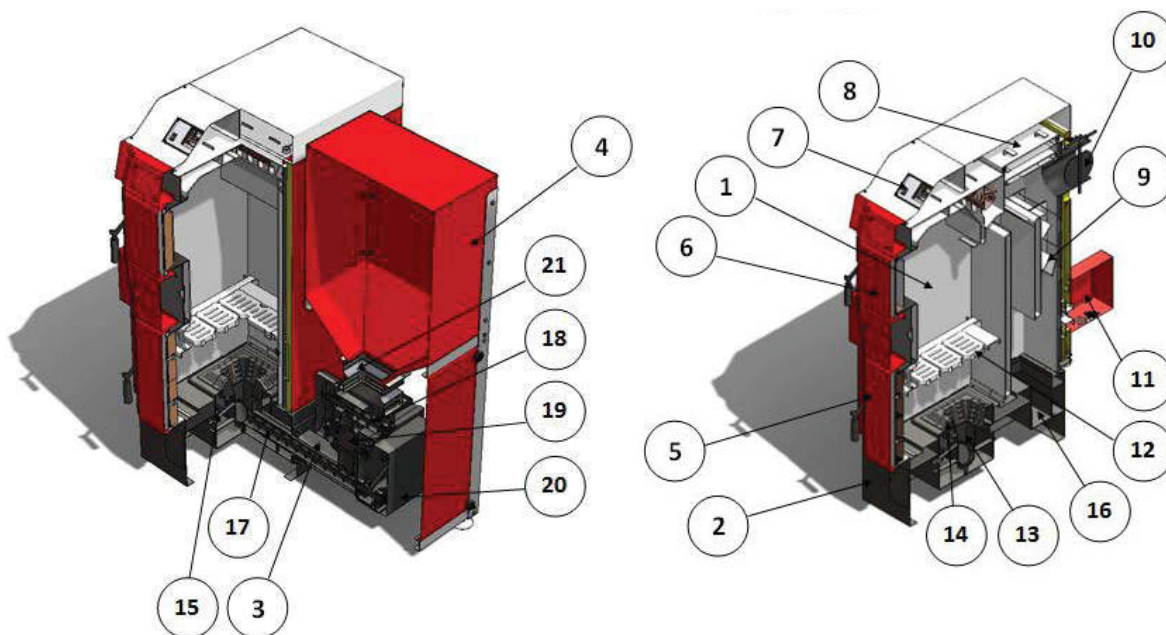
Разрез котла TKAN 1-2
